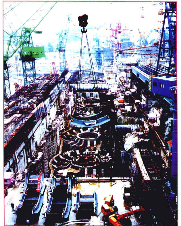
特大型水轮发电机组安装
