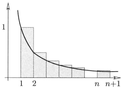
在函数 f(t) = \frac{1}{t} 上面的阶梯
