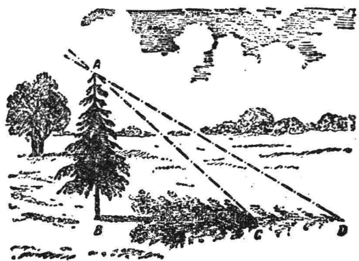
图3. 半影是怎样形成的？
