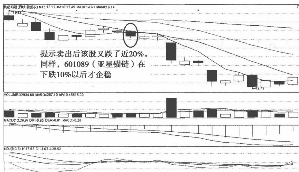
图 1-2 601177 的走势
