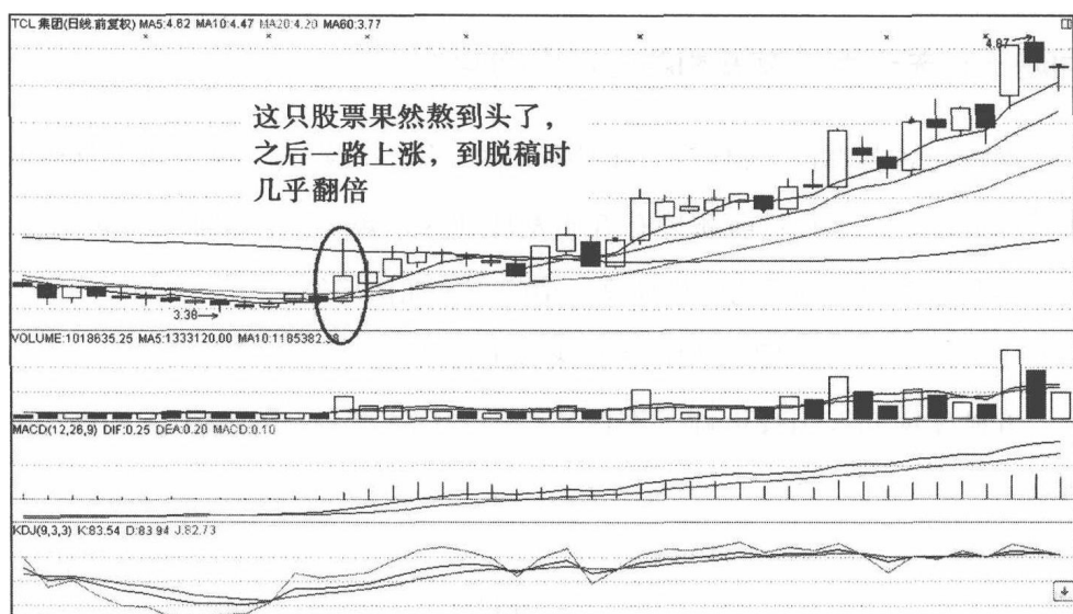
图 1-1 000100 的走势
