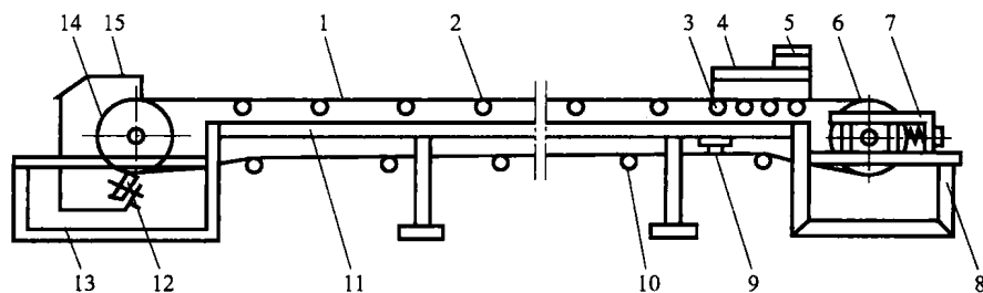
图 1-1-1 带式输送机
