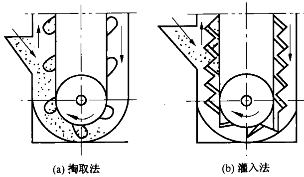
图 1-1-11 斗式提升机的装料方式
