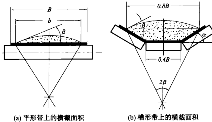
图 1-1-9 物料在输送带上的横截面积
