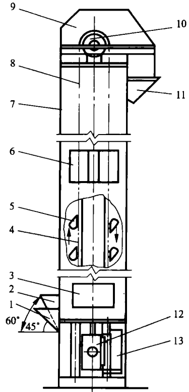
图 1-1-10 斗式提升机
