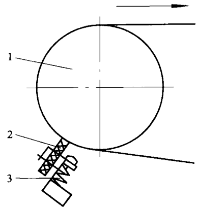
图 1-1-8 弹簧清扫器安装图 1—滚筒; 2—刮板; 3—弹簧
