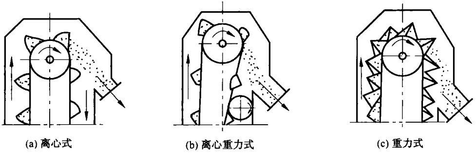
图 1-1-12 斗式提升机的卸料方式
