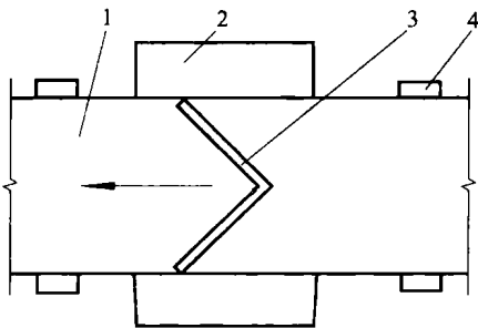
图 1-1-6 刮板卸料器
