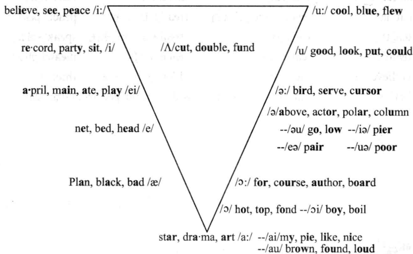
图 1-1 元音发音口形大小对比示意图
