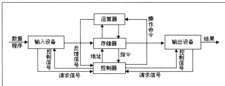
图 1-1 计算机的结构
