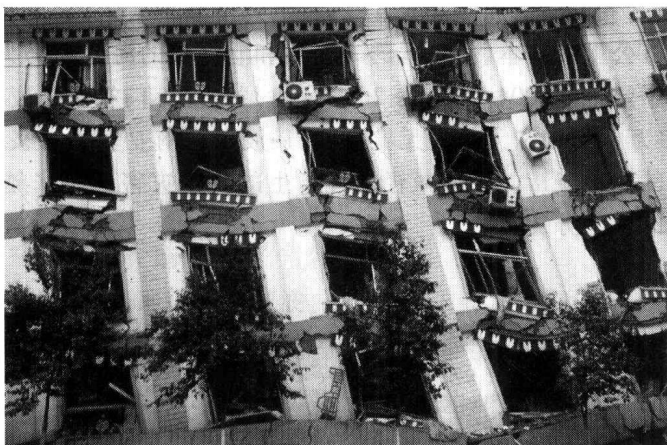
图 1-11 结构塑性变形引起的破坏
