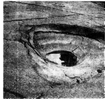
图 1-6 喷砂冒水
