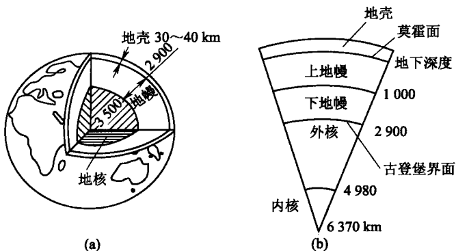
图 1-1 地球的构造
