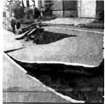
图 1-4 日本新潟地震后地路上地裂缝
