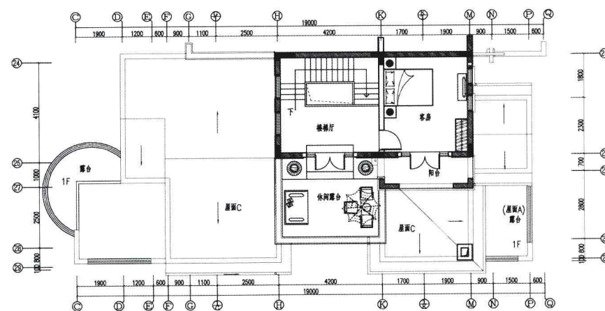
三层平面图
