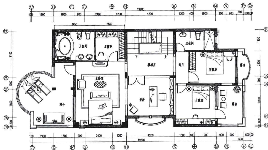
二层平面图
