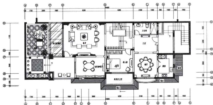
一层平面图
