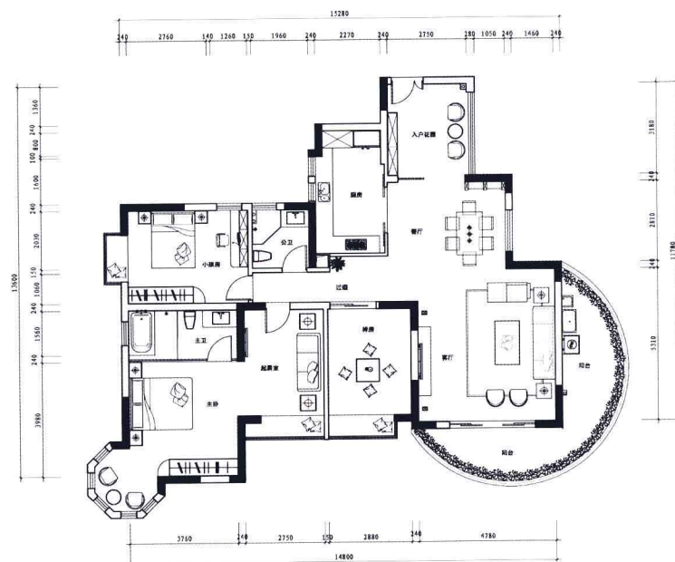
平面图
