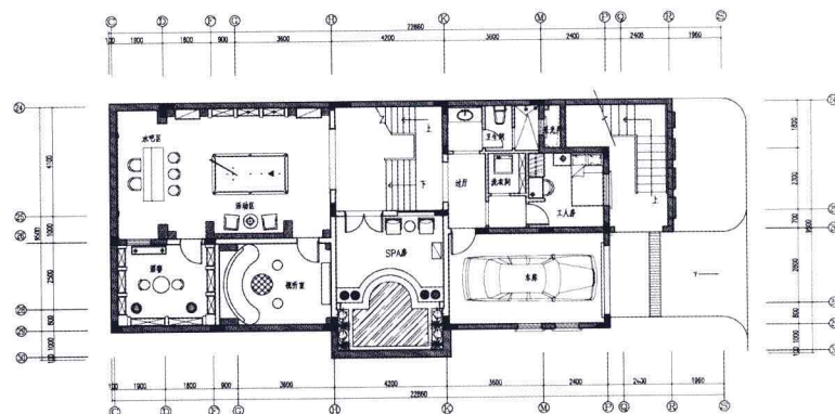
地下一层平面图
