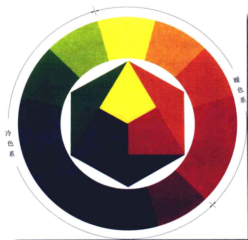
彩图10 色轮
