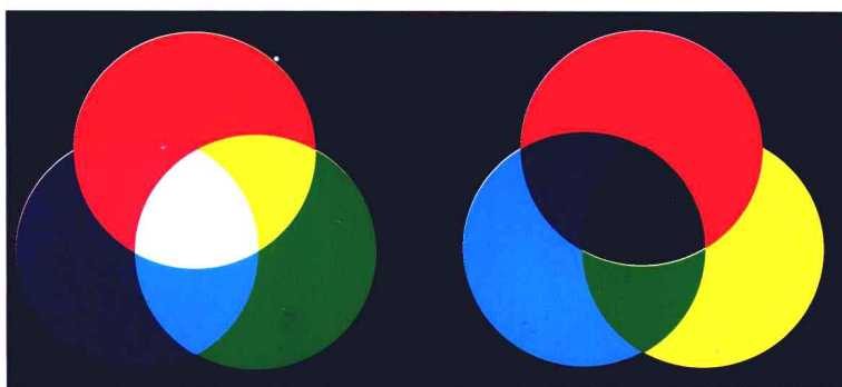
彩图8 三原色
