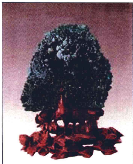
彩图1 孔雀石
