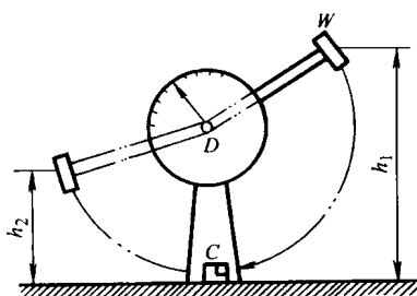
图 2-4 冲击韧度的测定方法
