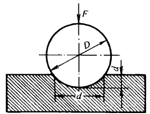
图 2-2 布氏硬度试验法
