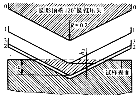
图 2-3 洛氏硬度试验法
