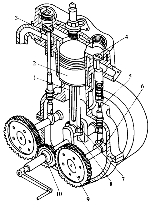
图 1-2 单缸内燃机构造
