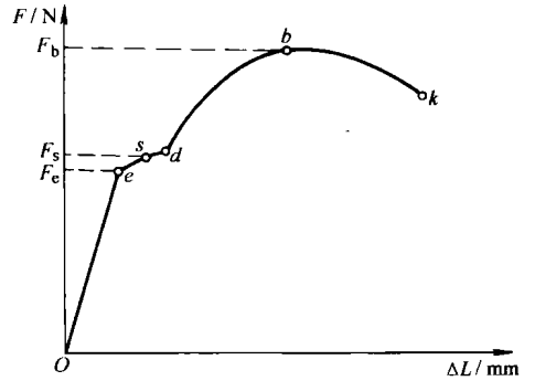
图 2-1 低碳钢的拉伸曲线
