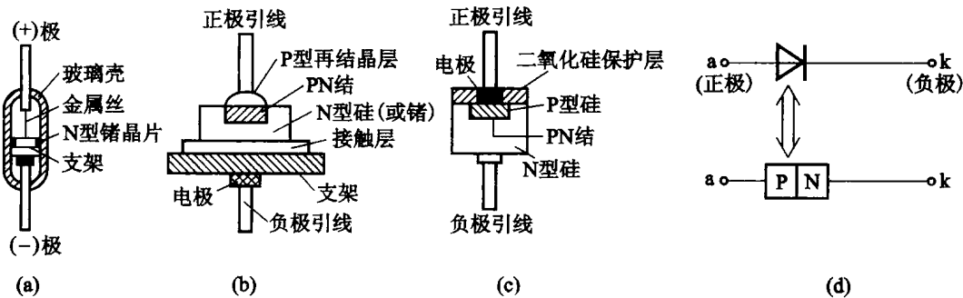
图 1-2 二极管的结构类型及符号 (a) 点接触型 (b) 面接触型 (c) 平面型 (d) 符号
