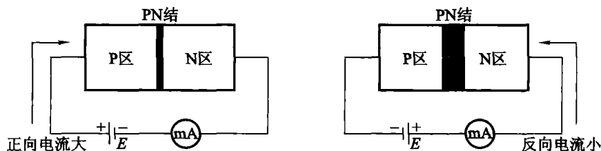
图 1-1 PN 结的单向导电性
