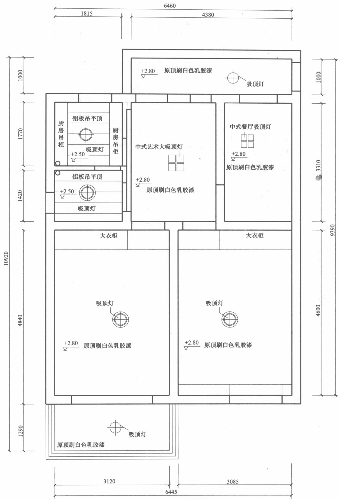
总顶平面规划图
