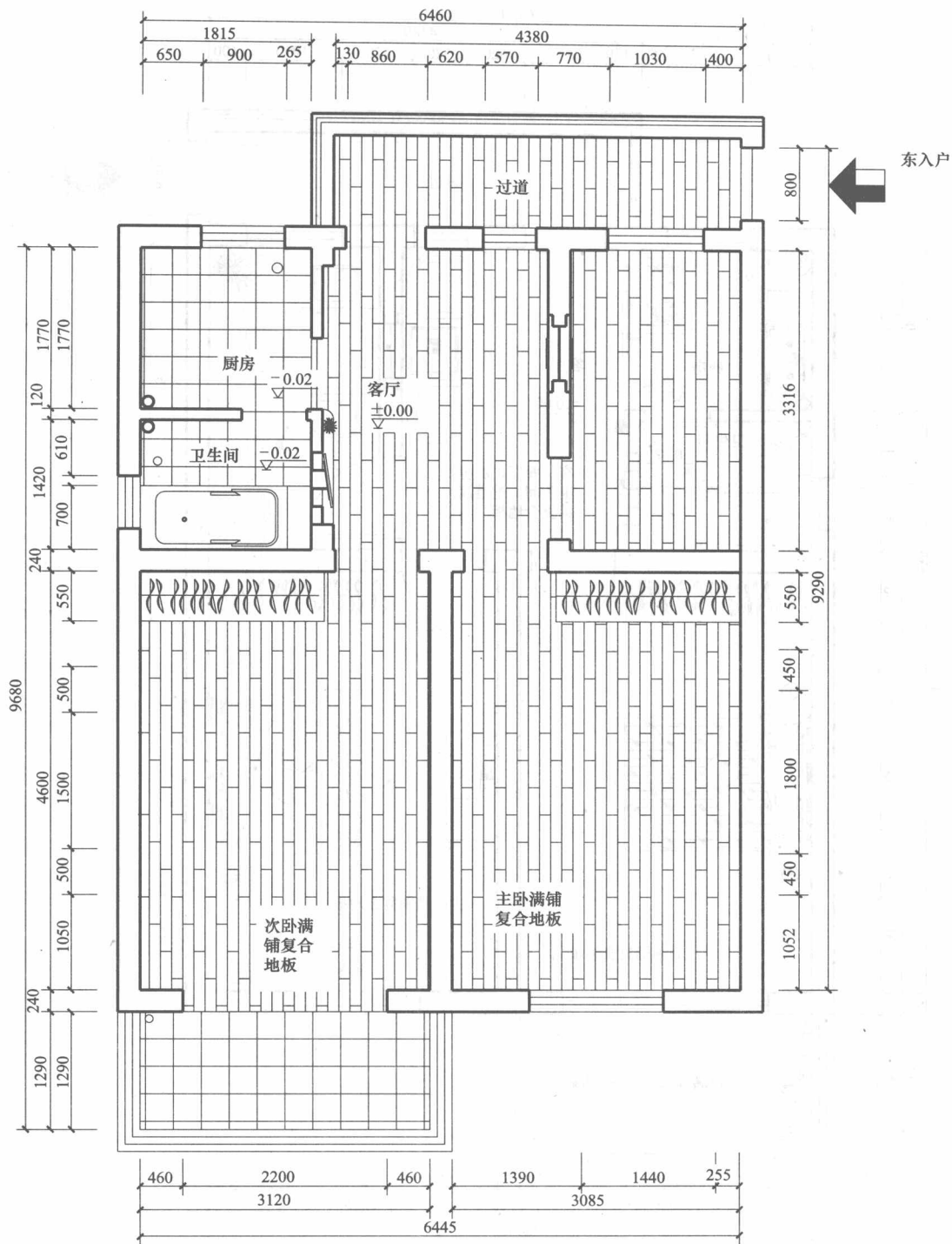
地面铺贴图
