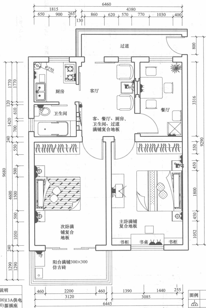
插座布置图
