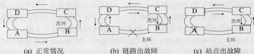
图 1-2 具有双环的 FDDI
