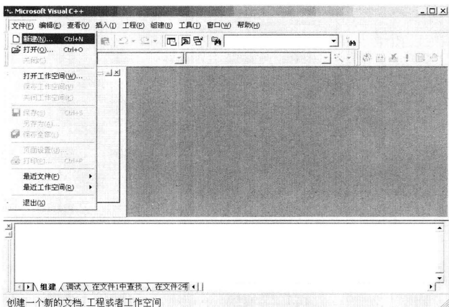
图 1-3 新建源文件
