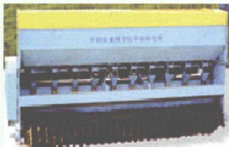
彩图2-1 2BC-10型苜蓿草种籽播种机
