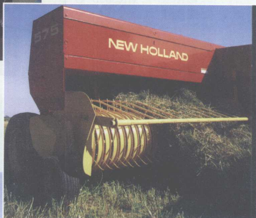
彩图 6-13 纽荷兰 小方捆打捆机
