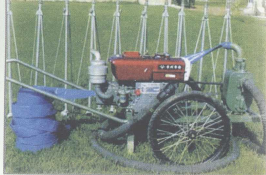
彩图 3-2 柴油机 自吸泵喷灌系列
