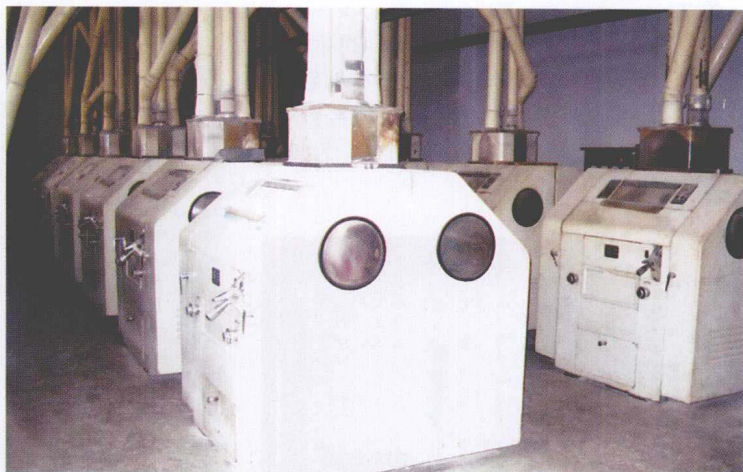
磨粉机设备
