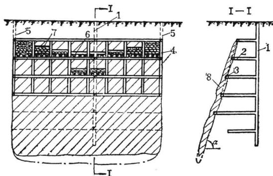
图 1-8 矿床开采步骤和三级储量图
