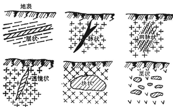
图 1-3 矿体的形状
