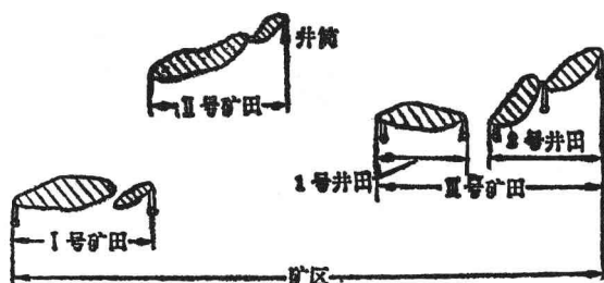
图 1-4 矿区、矿田和井田
