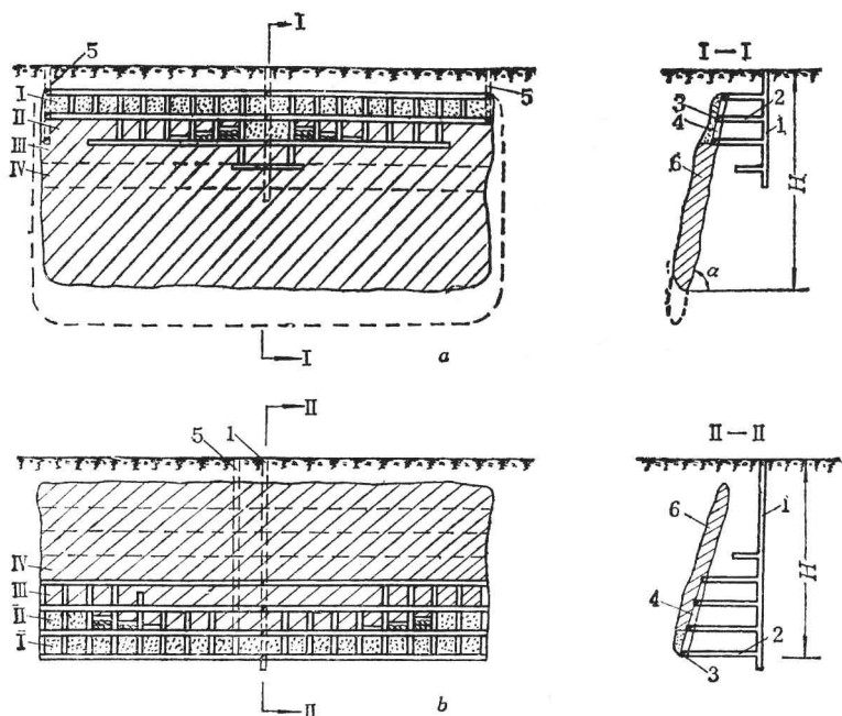
图 1-7 井田中的开采顺序
