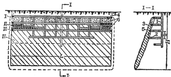
图 1-5 阶段与采区的划分图
