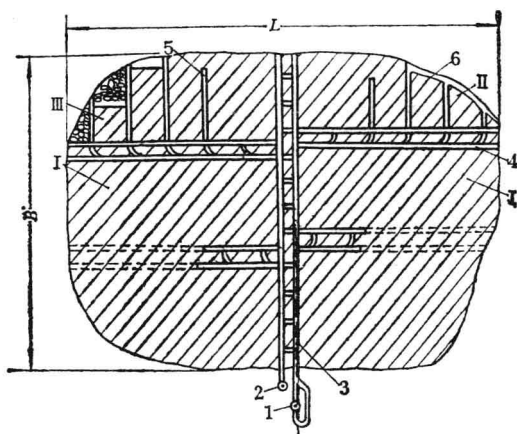
图 1-6 盘区与矿壁的划分图
