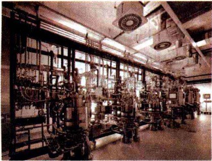
图3 发酵罐
