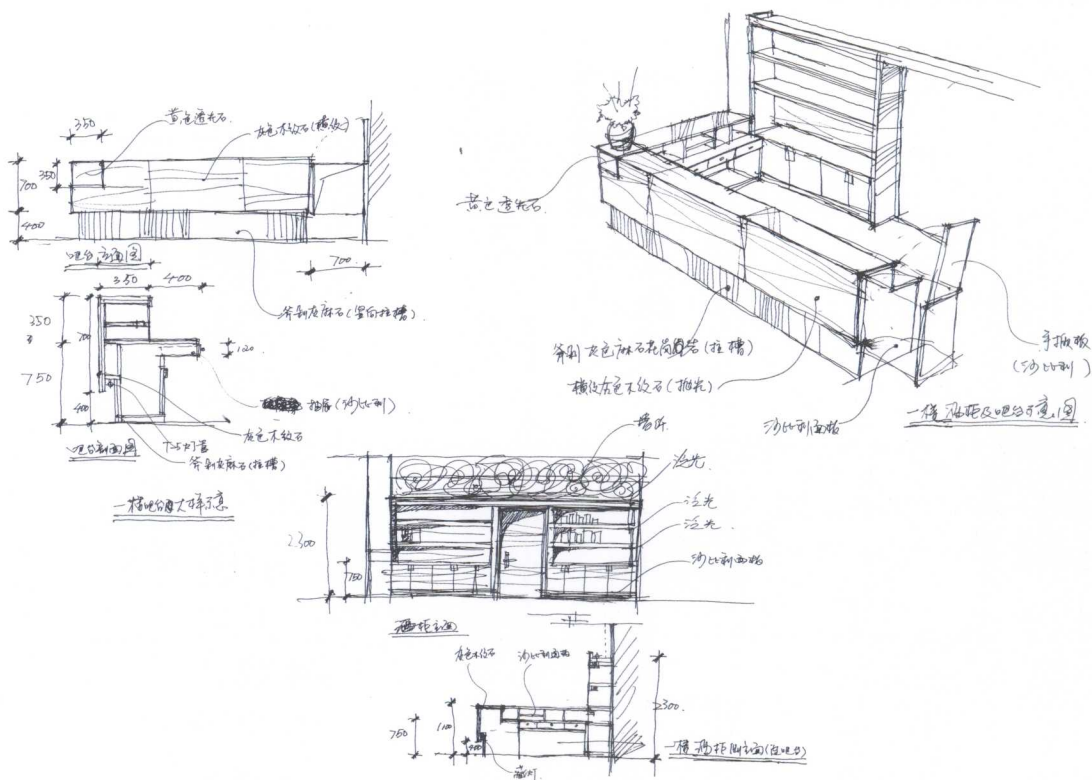
▲某酒吧酒柜设计草图 / 杨健
