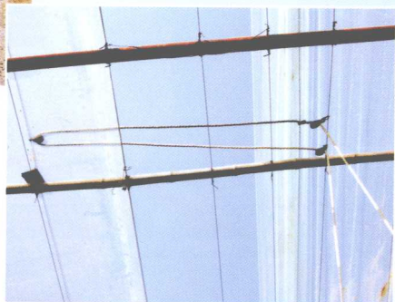
冬暖大棚天窗通风操作系统
