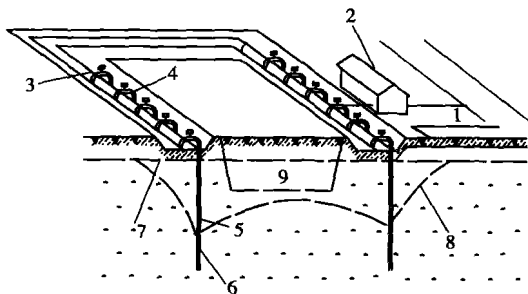
图 1.3 轻型井点降低地下水位示意
