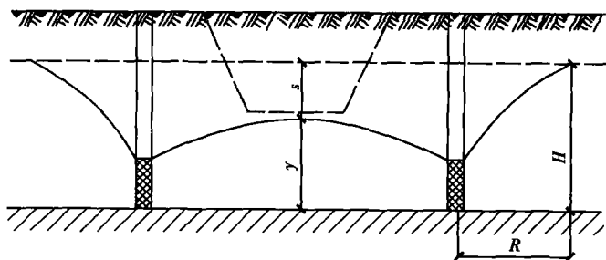
图 1.13 无压环状完整井
