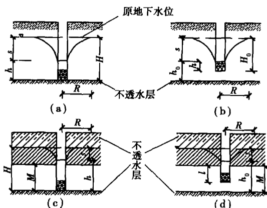
图 1.11 水井的分类
