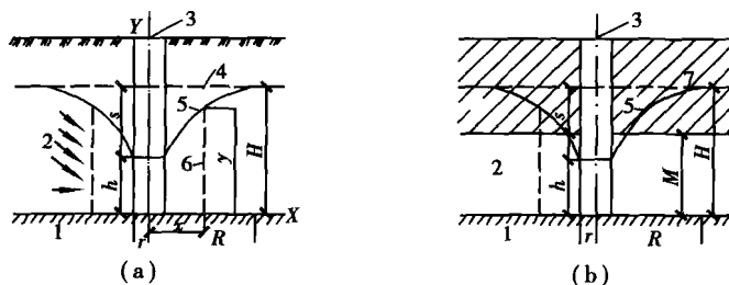
图 1.12 完整井水位降落曲线
