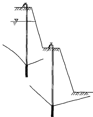
图 1.10 二级轻型井点
