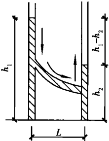
图 1.1 土的渗流实验
