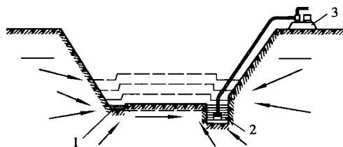
图 1.2 集水井降水
