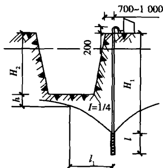
图 1.9 高程布置
