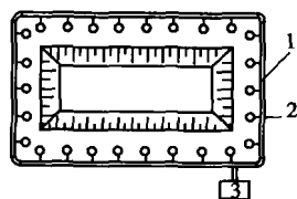
图 1.8 环形井点的布置
