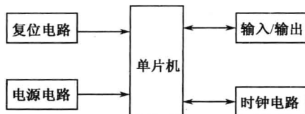
图 1-3 单片机最小系统结构示意图
