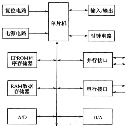
图 1-4 单片机扩展系统结构示意图
