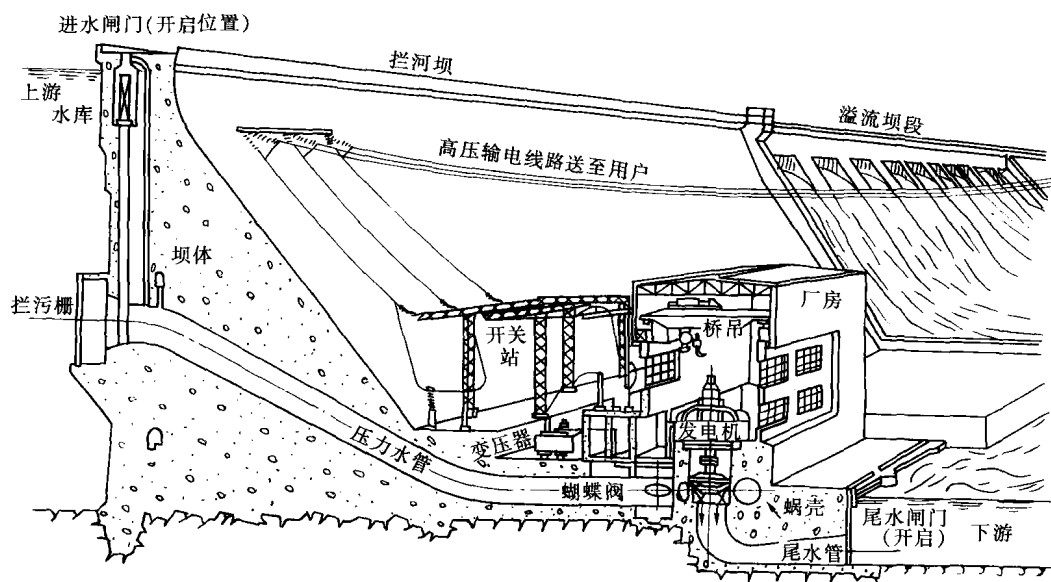
图 0-3 水力发电厂生产过程示意图
