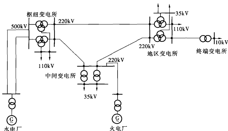
图 0-5 降压变电所类型示意图
