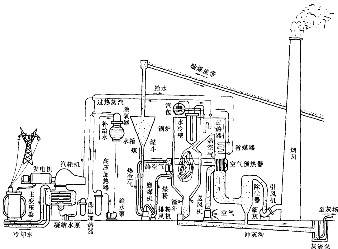
图 0-2 凝汽式火力发电厂生产过程示意图
