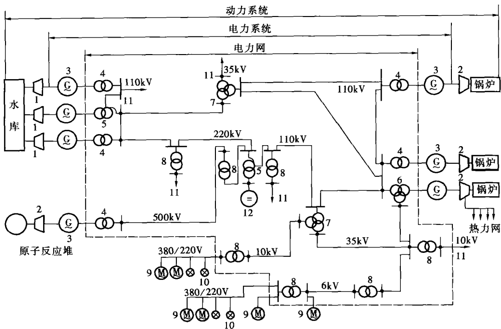
图 0-1 动力系统、电力系统、电网的示意图
