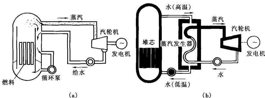
图 0-4 原子能发电厂生产过程示意图
