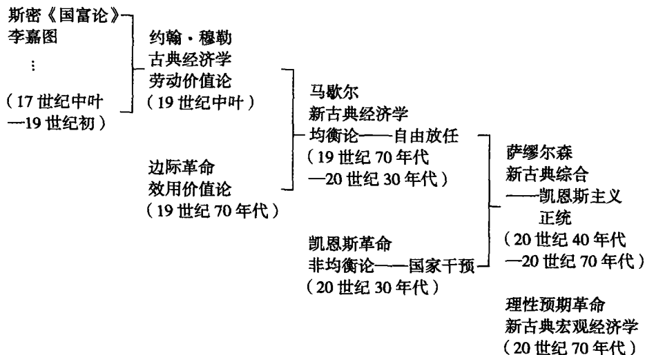
图 1—1 西方经济学发展历程图
