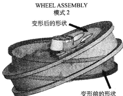
图 1-2 变形前后的形状对比
