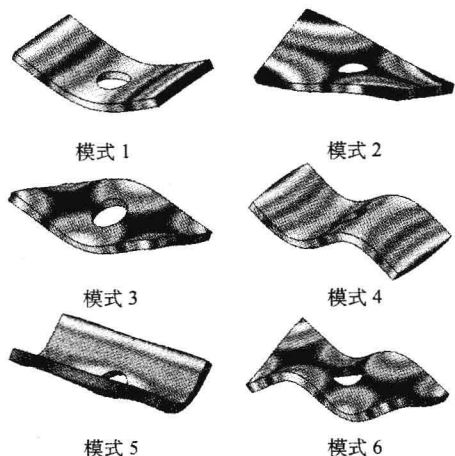
图 1-1 带孔无支撑平板的几种模式
