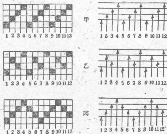
图 3-7 穿綜圖
