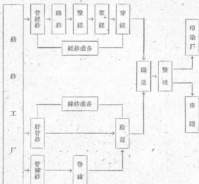
图 3-2 一般的織造工艺过程
