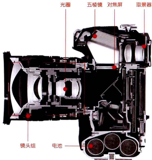
» 数码单反相机剖面图
