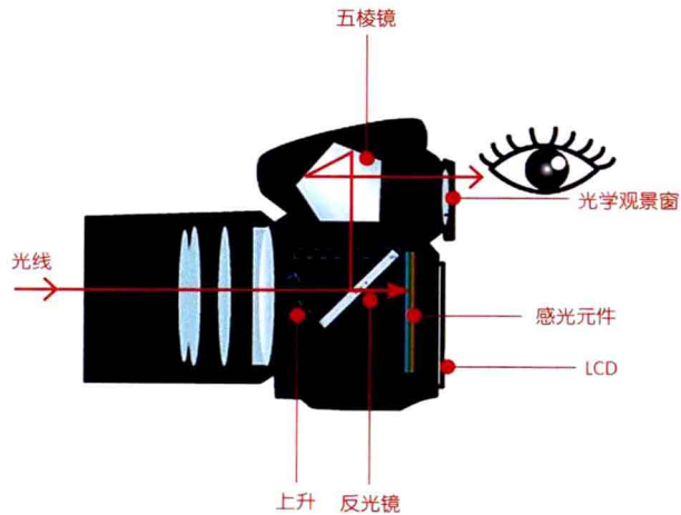
» 单反相机中的光线走向图
