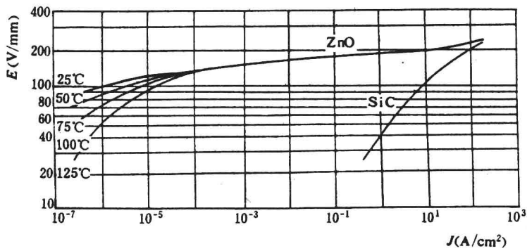
图 2-5 MOV的温度响应特性
