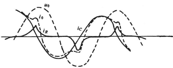
图 2-3 在工频低电压作用下MOV的电压、电流波形
