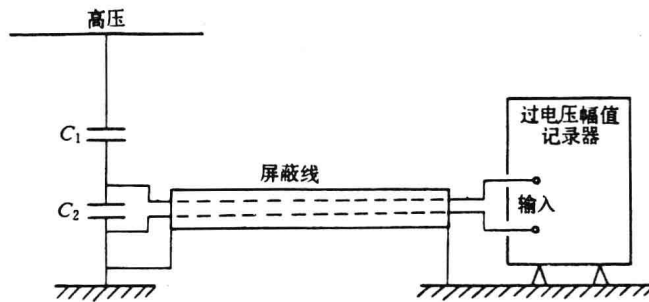
图 1-2 过电压幅值记录器的接入
