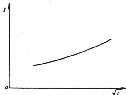
图 2-7 MOV 在长期持续电压作用下电流与时间的关系
