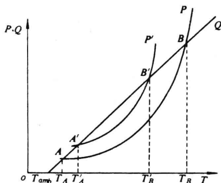
图 2-10 MOA的热平衡
