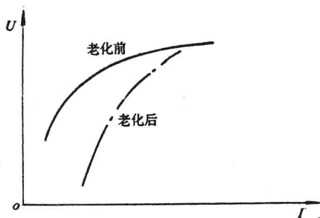
图 2-6 MOV 老化前后的伏安特性
