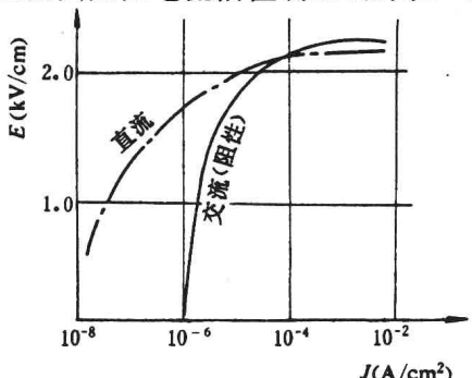
图 2-4 MOV的直流和交流 E-J 特性
