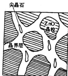
图 2-1 \text{ZnO} 电阻片显微结构
