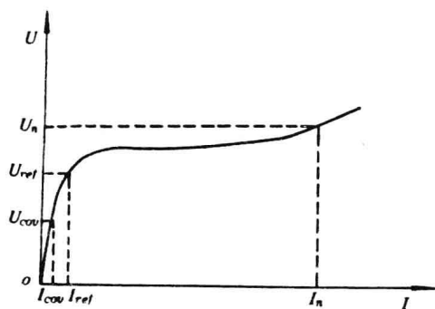
图 2-9 无间隙MOA的伏安特性
