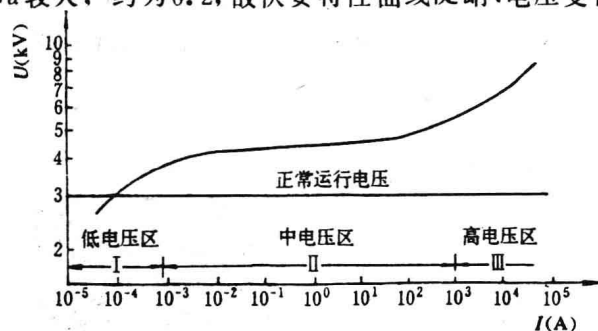
图 2-2 MOV的全伏安特性曲线
