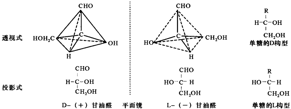
图 1-2 甘油醛的对映体及单糖的 D 与 L 构型
