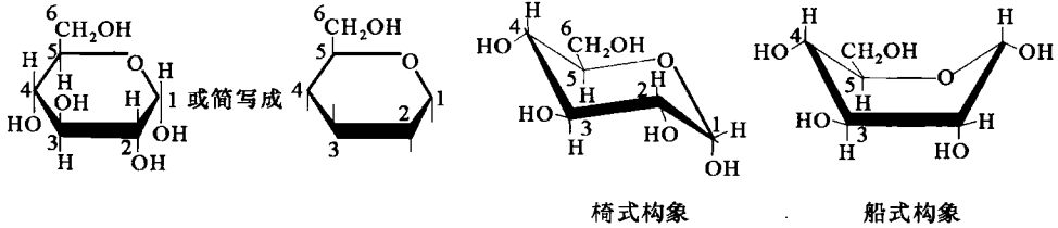
图 1-3 葡萄糖透视式环状结构和 \alpha -D-葡萄糖的椅式、船式构象
