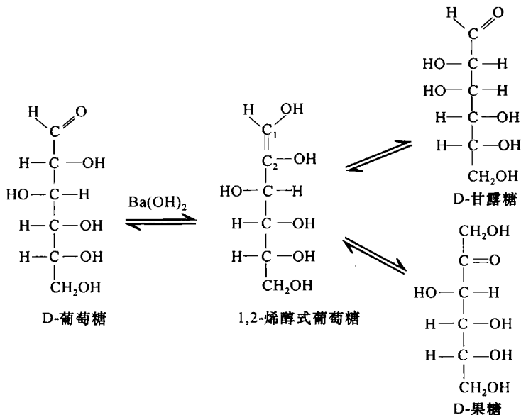
图 1-5 单糖在碱催化下的酮—烯醇互变异
