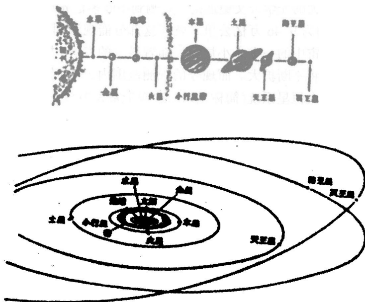
图 4-2 太阳系及行星示意图
