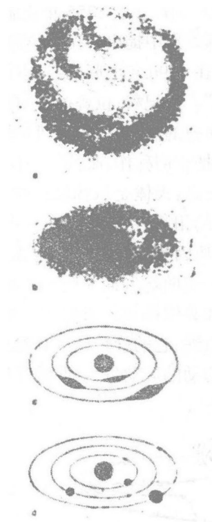
图 4-4 康德——拉普拉斯星云假说图示
