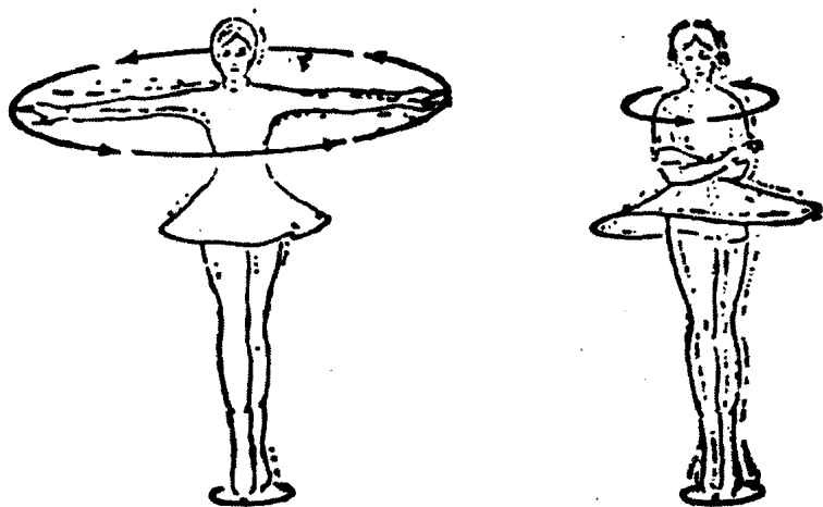
图 4-3 角动量守恒示意图。
