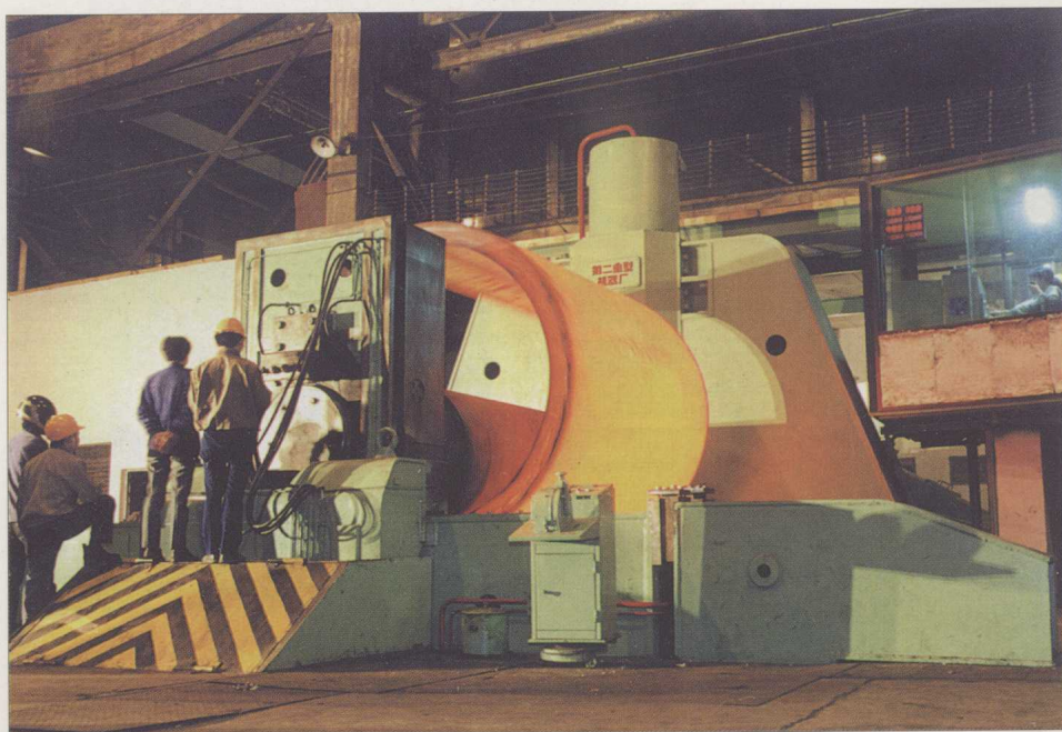
杭州锅炉厂生产的具有 80 年代先进水平的重型三辊卷板机
