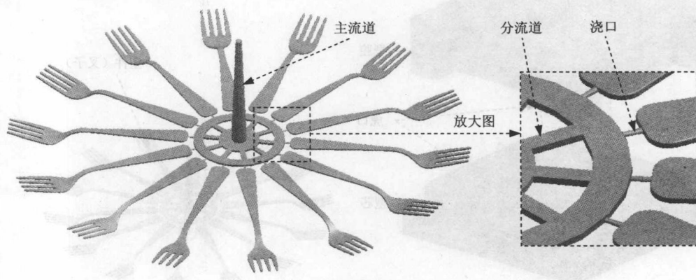
图 1.1.5 浇注系统
