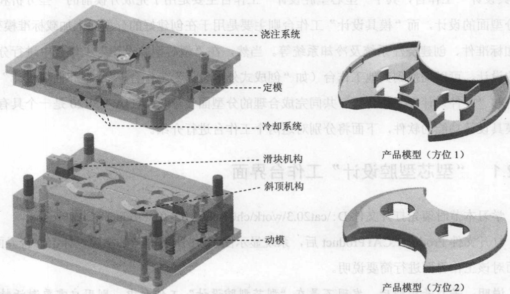
图 1.1.6 模架设计
