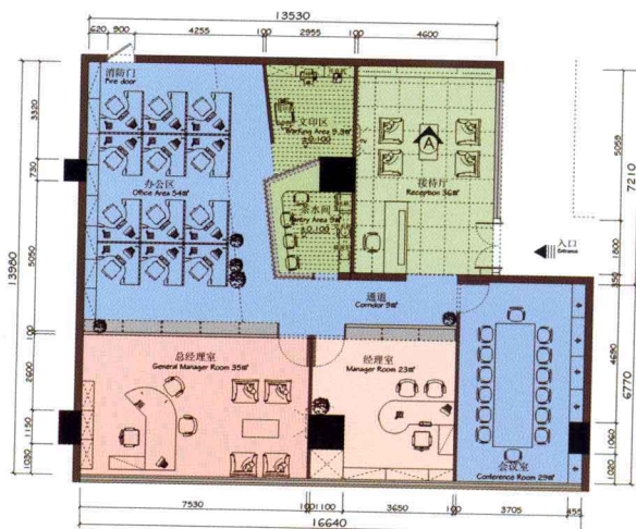
平面图
