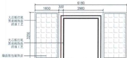
形象墙A立面图
