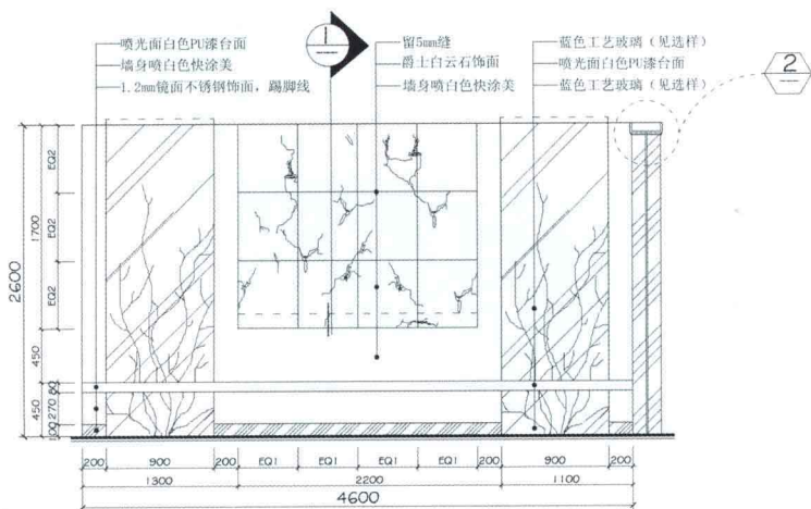
接待厅①立面图
