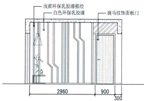
休息区B立面图
