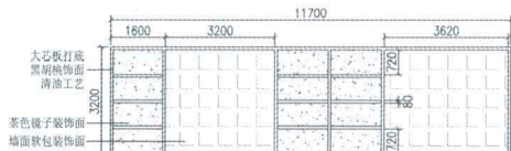
形象墙B立面图
