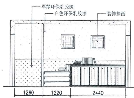
阅读区D立面图
