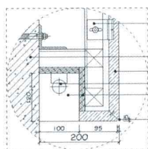
接待厅①剖面大样图
