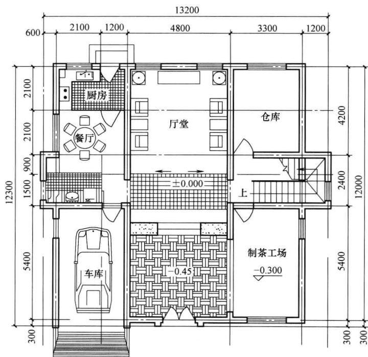
一层平面图
