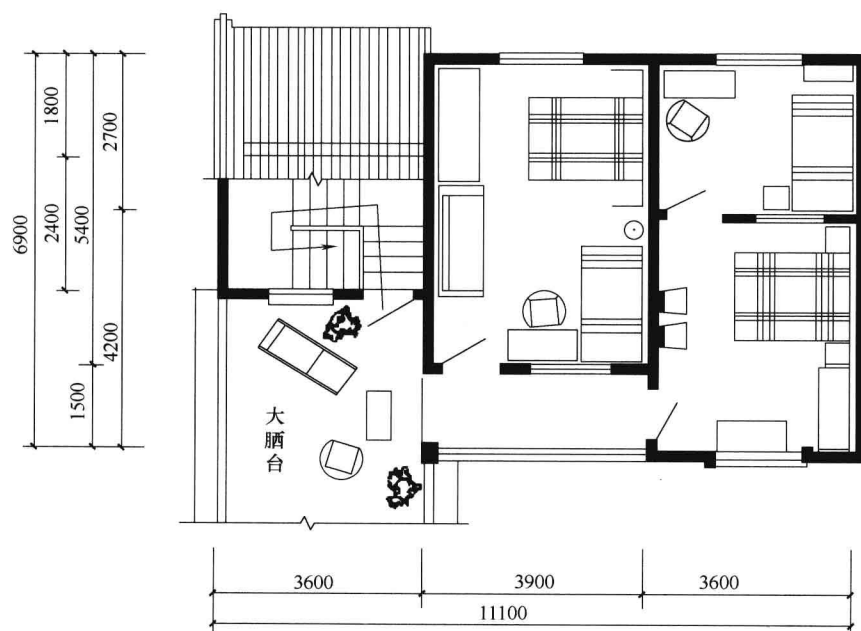
二层平面图
