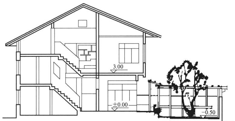
A—A剖面图
