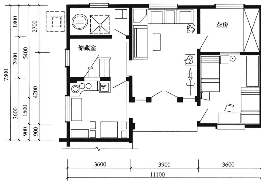
一层平面图
