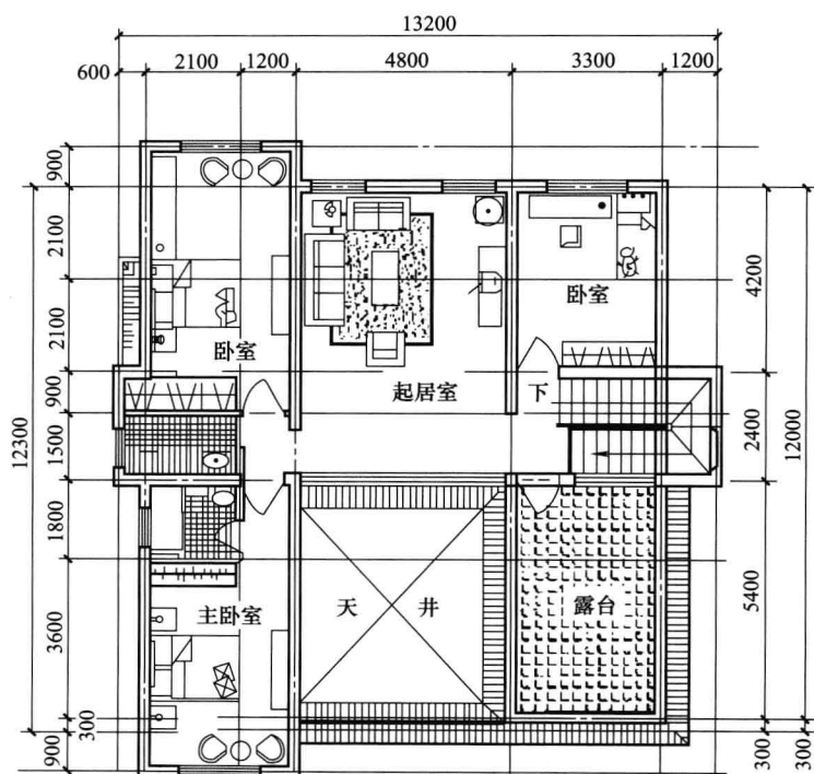
二层平面图
