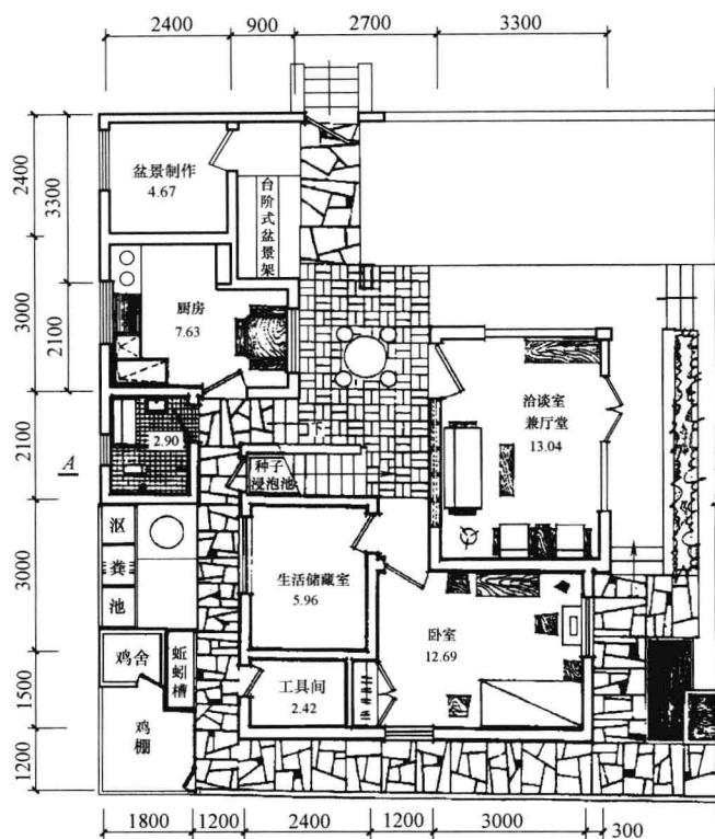
一层平面图
