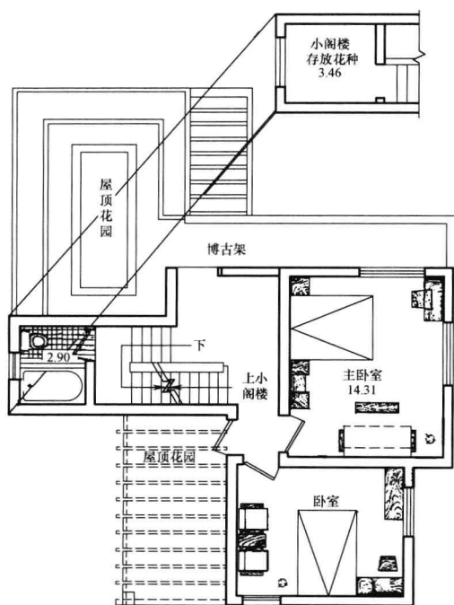
二层平面图
