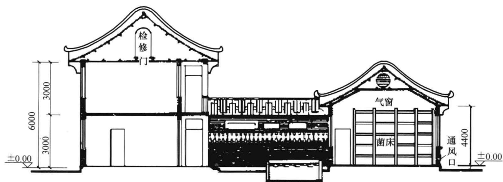
I—I剖面图
