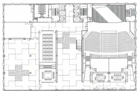
7 层平面图
