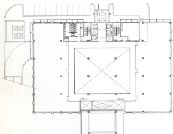
1 层平面图
