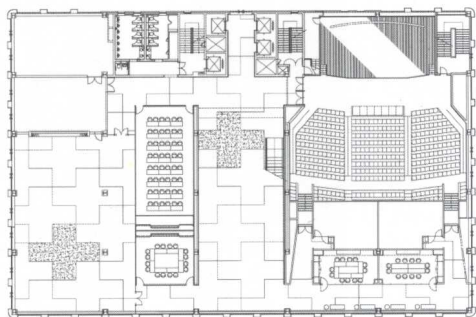
8 层平面图
