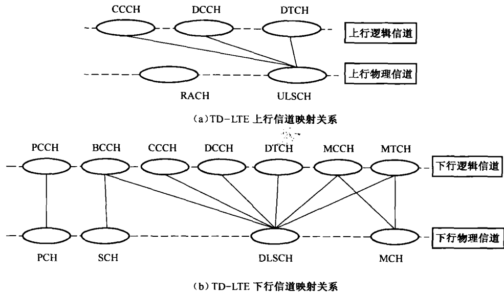
图 1-2 TD-LTE 系统中上、下行信道映射关系
