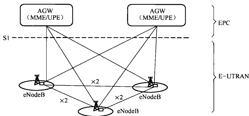
图 1-1 LTE 网络架构图
