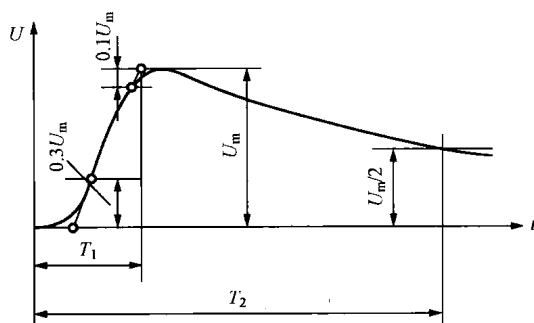
图 1-8 标准冲击全波的波形图
