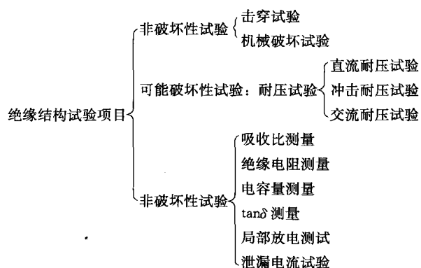
图 1-3 绝缘结构的试验项目分类图
