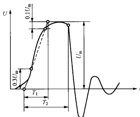
图 1-9 标准冲击截波波形
