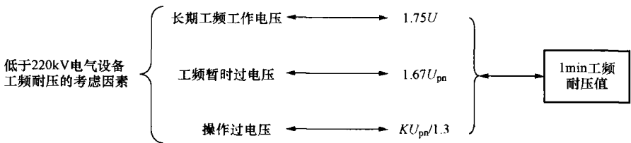
图 1-11 低于 220kV 的电气设备工频电压的确定因素
