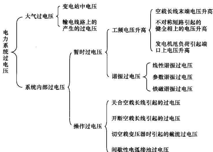
图 1-7 电力系统各种过电压
