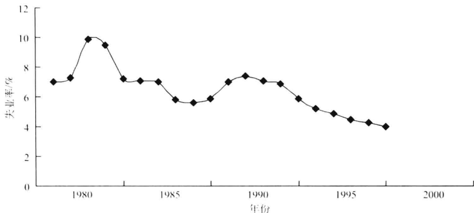
图 1-1 1980~2000 年美国的两次失业高峰
