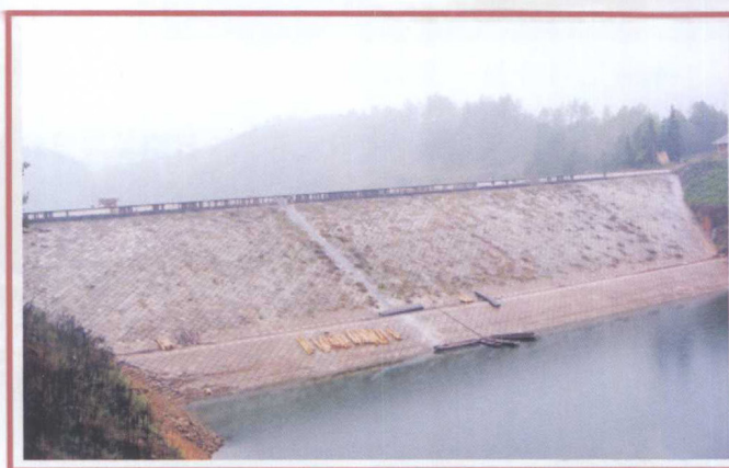
黎平墨门山大坝
