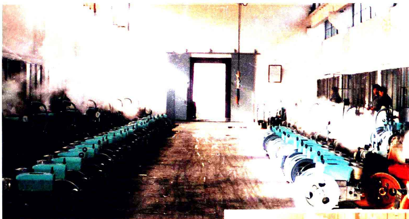
▲ 扬州市动力机厂 S195 柴油机测试车间
