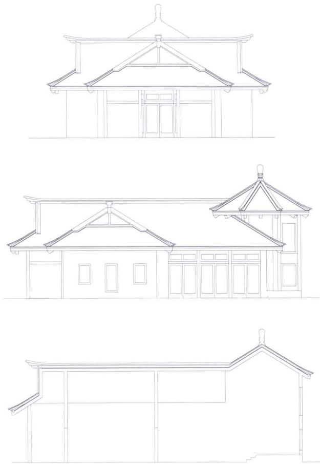
婚礼亭剖立面
