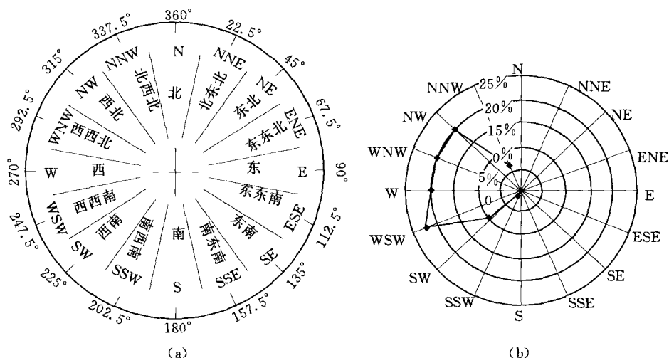
图 1-1 风向表示法 (a) 风向 16 方位图；(b) 风向玫瑰图
