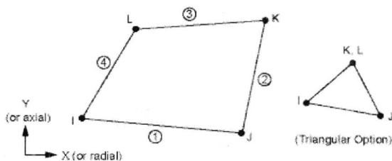
图 2-1 FLUID141 的几何形状
