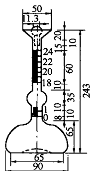
图 1-1 李氏瓶
