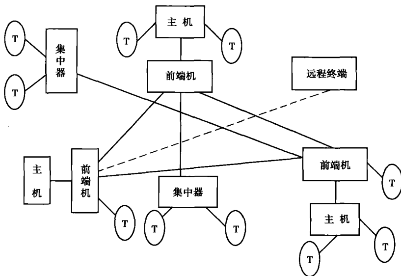
图 1.2 分组交换网的示意图
