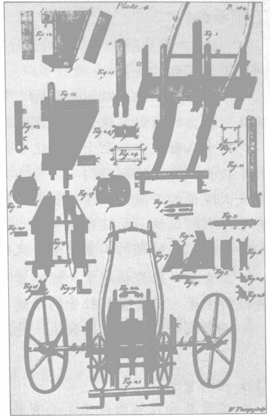
塔爾發明的種子條播機
