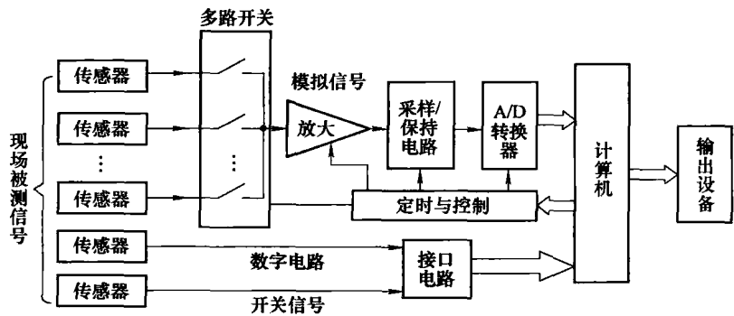
图 1-3 基本型现代检测系统
