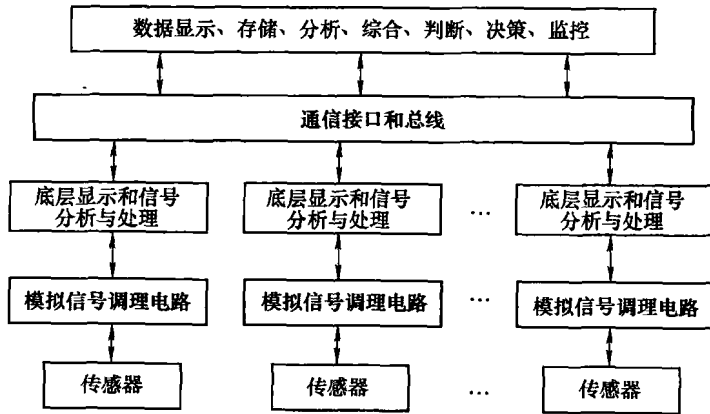
图 1-2 检测系统的一般组成框图
