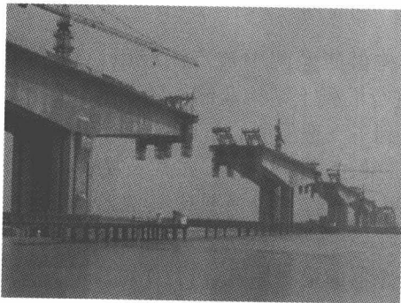
图 1.3 山东滨州黄河大桥光纤光栅监测系统 [13] 图 1.4 悬臂施工阶段的广阳岛大桥主桥 [14]
