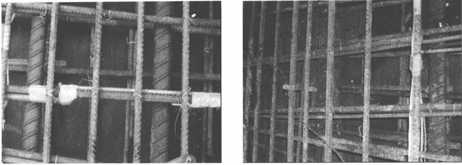
图 1.5 重庆广阳岛大桥光纤光栅传感器布设 [14]
