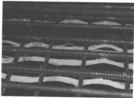
图 1.2 山东滨州黄河大桥光纤光栅传感器布设 [13]
