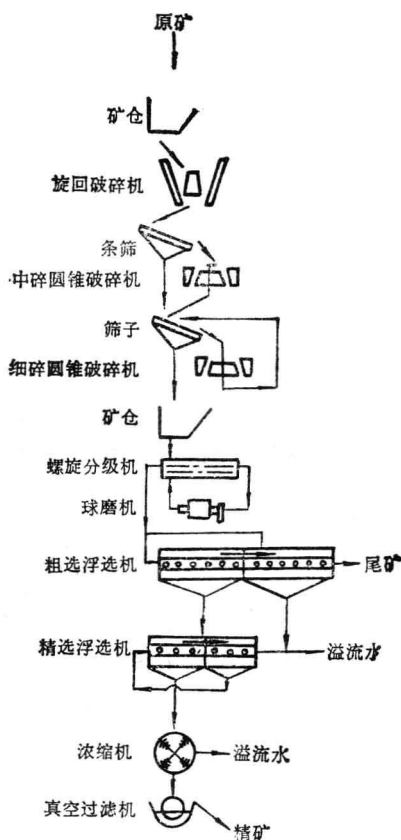
图 0-2 机械流程图
